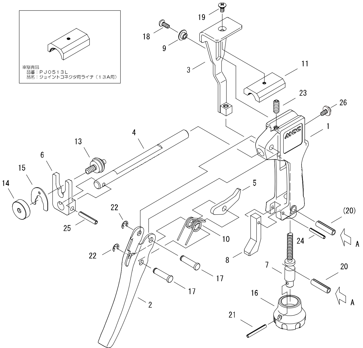
PJ-05 (ジョイントコネクタ)
