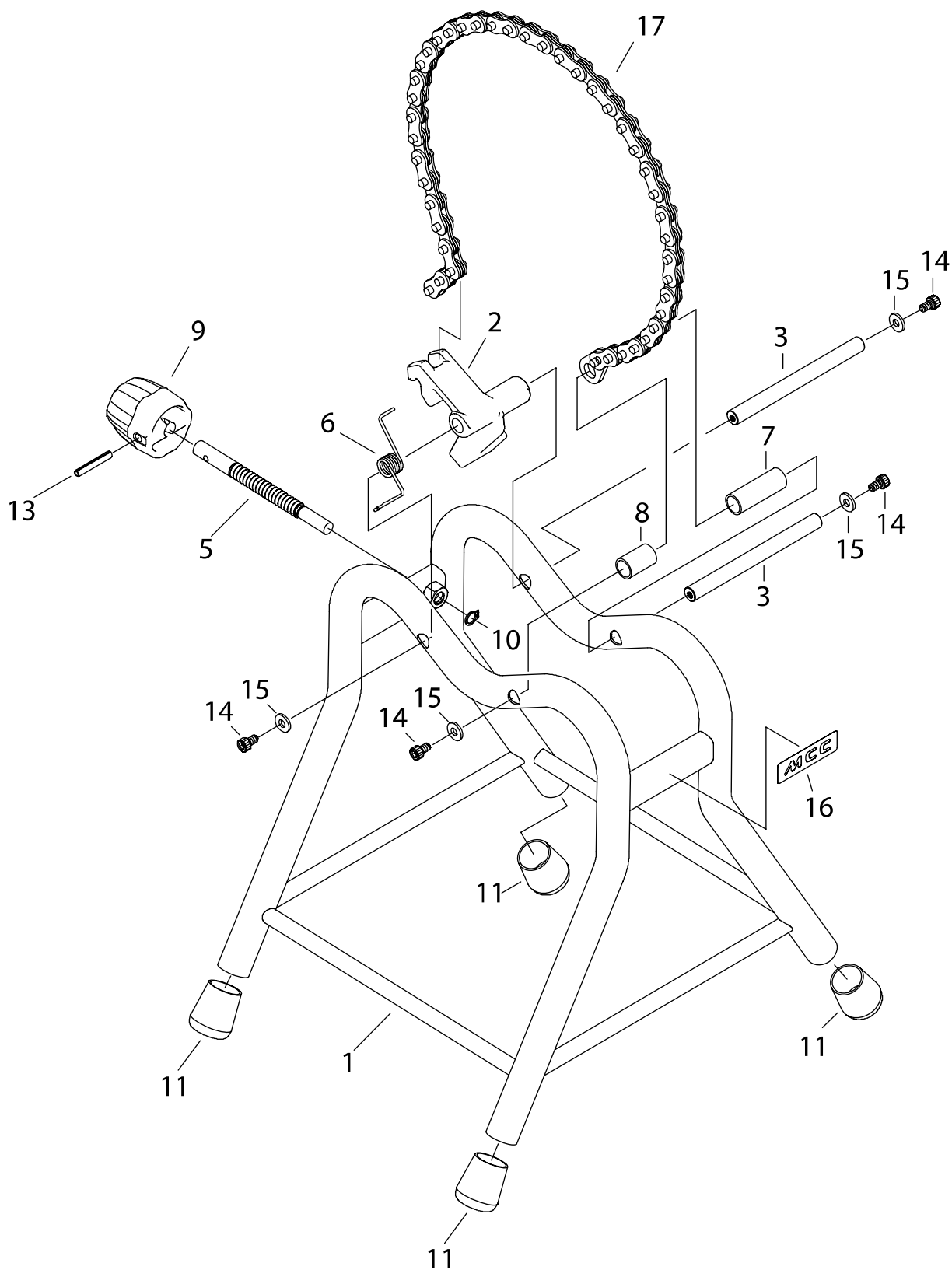
JPVS-250 (樹脂管バイスタンダード)
