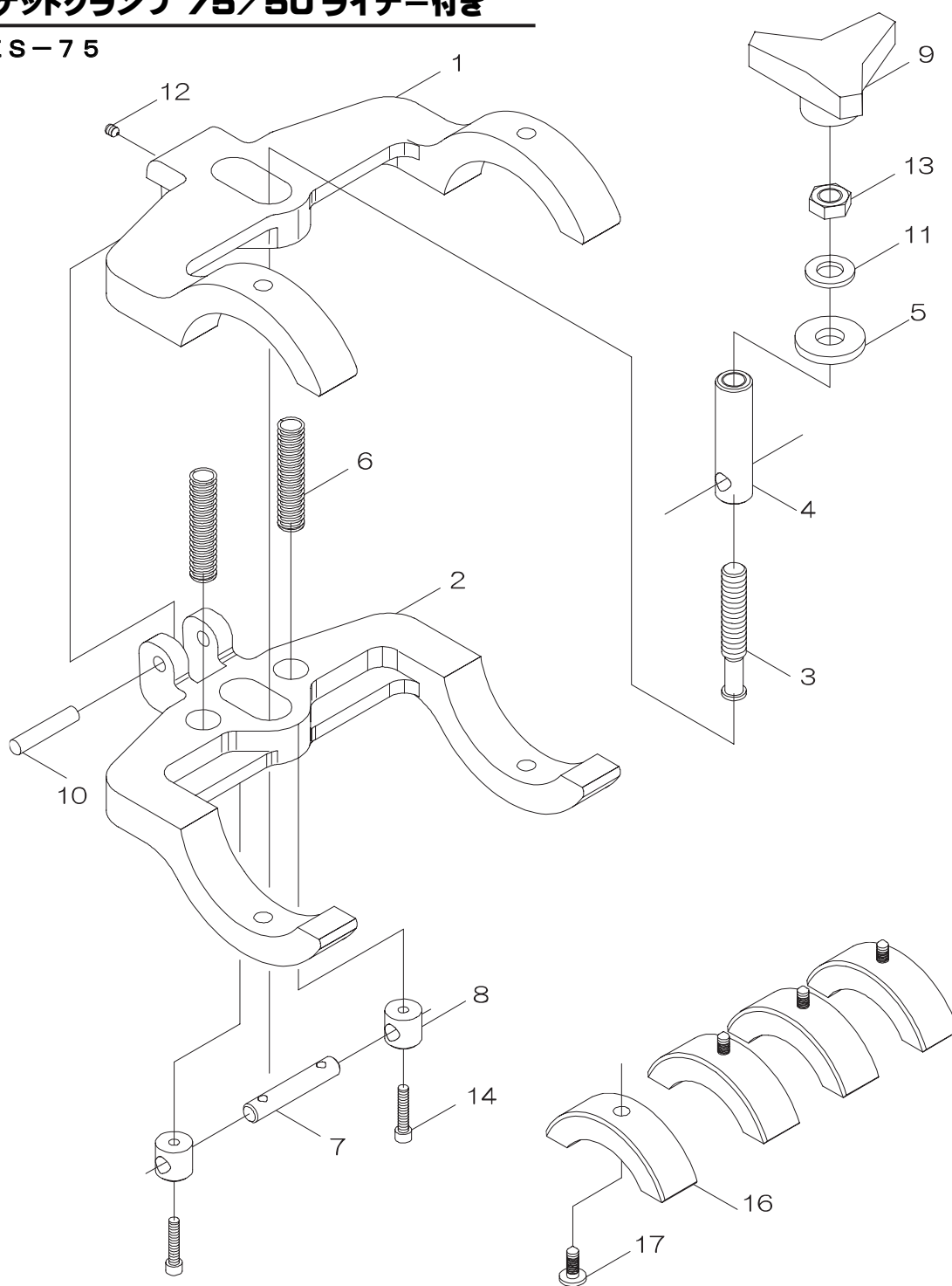
ES-75 (ソケットクランプ 75/50ライナー付き)
