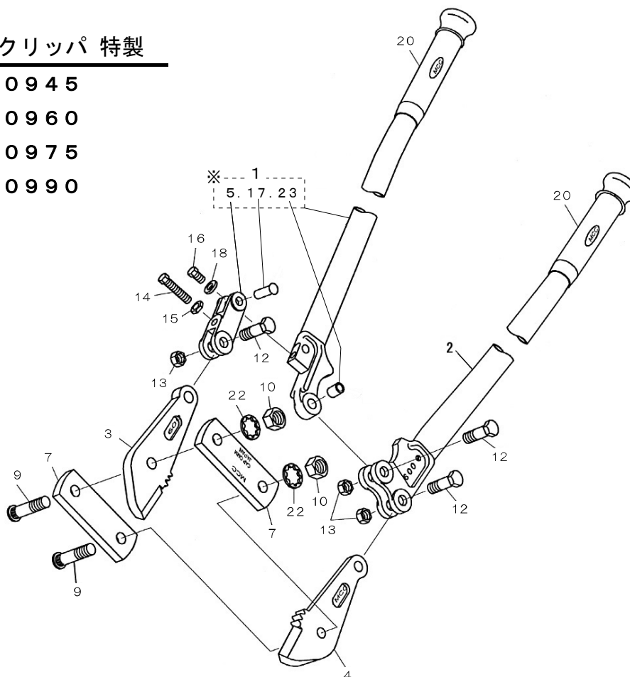
BC-0945 (ボルトクリッパ 特製 450)
