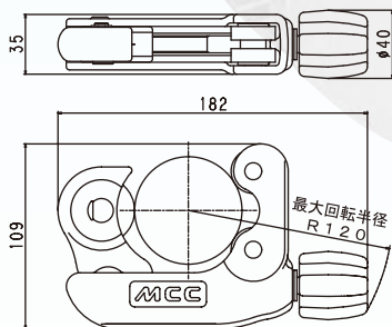
■ 寸法図 (単位:mm)
